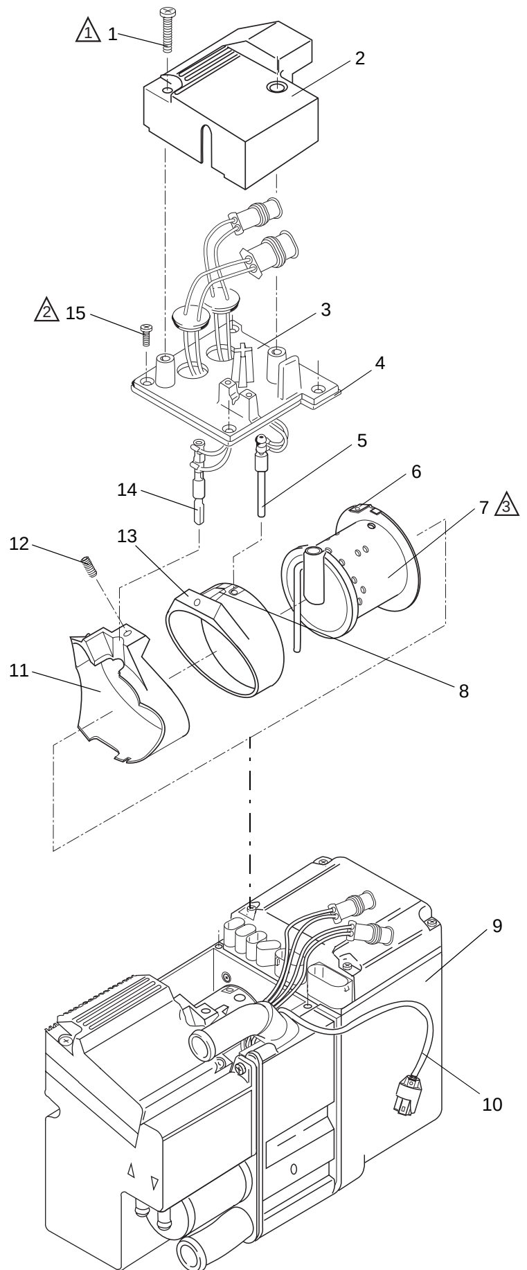
Abb. 809 Wechsel des Brennereinsatzes (Seite 1 von 2)
