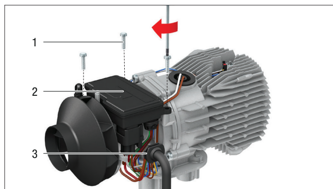
1 Крепежные винты M4 x 16 (Torx) 2 Блок управления 3 Втулка для кабельного жгута
