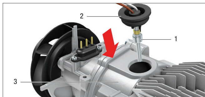
1 Электрод накаливания 3 Теплообменник 2 Резиновая втулка
