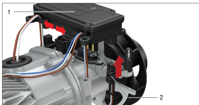
1 Блок управления 2 Штекер комбинированного датчика и датчика температуры
