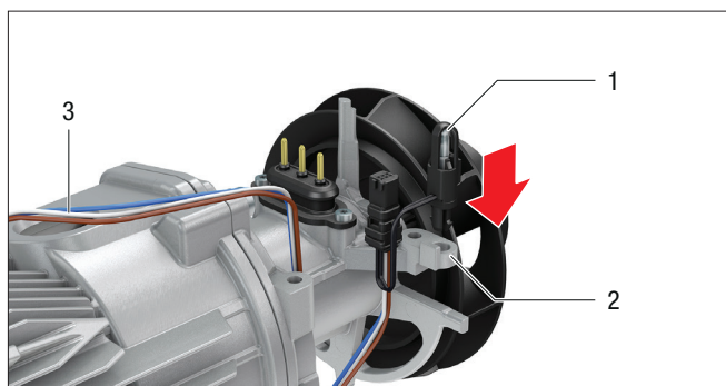
1 Датчик температуры 2 Гнездо датчика температуры 3 Соединительные провода
