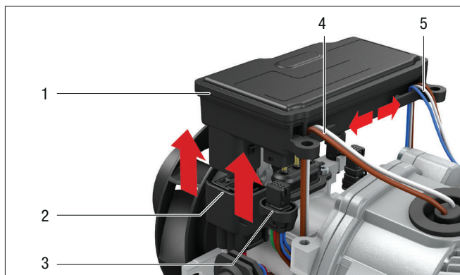
1 Блок управления 2 Штекер электропитания и электрода накаливания 3 Штекер кабельного жгута 4 Соединительные провода электрода накаливания 5 Соединительные провода комбинированного датчика
