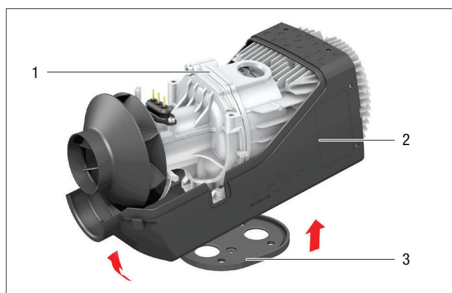
1 Отопительный прибор 3 Фланцевое уплотнение 2 Нижняя часть кожуха
