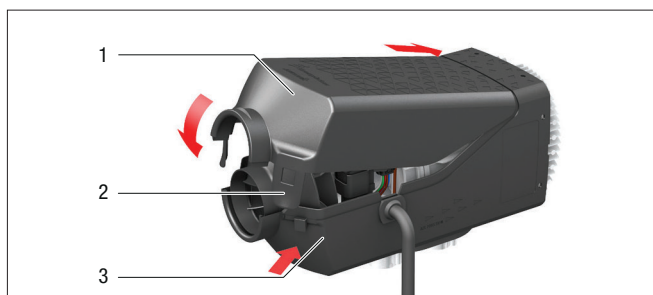
1 Верхняя половина кожуха 3 Нижняя часть кожуха 2 Фиксирующая защелка
